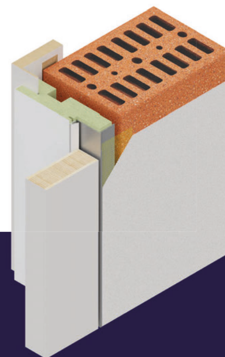
Ościeżnica do drzwi ukrytych
