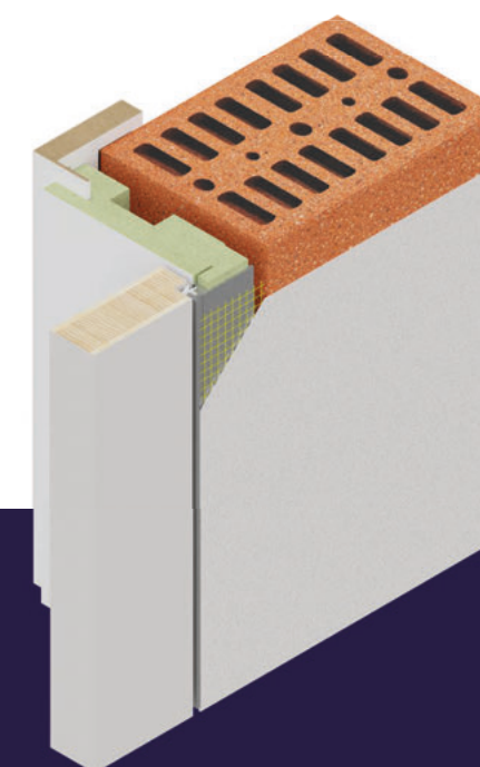
Ościeżnica do drzwi ukrytych rewersyjnych
